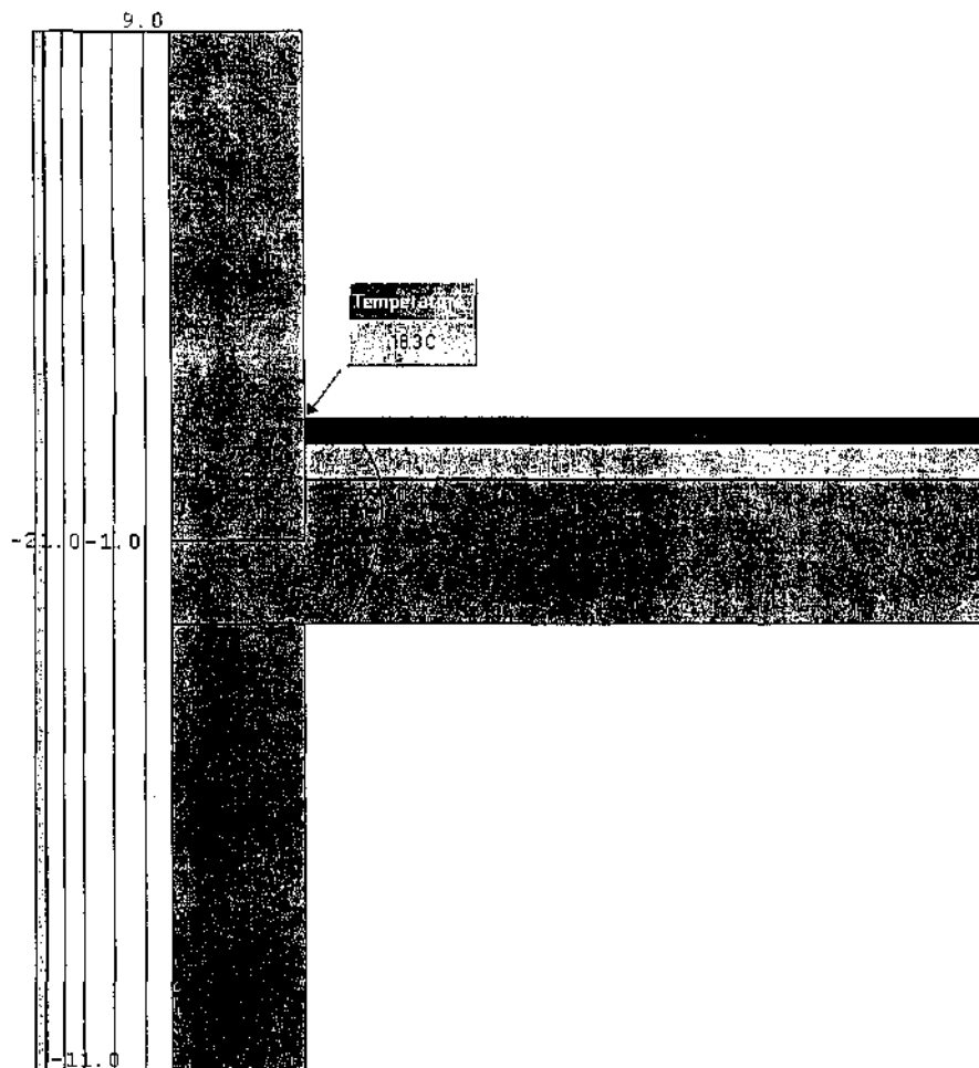
Рисунок А.3 – Температурне поле конструктивного рішення вузла примикання зовнішніх стін до плити покриття
