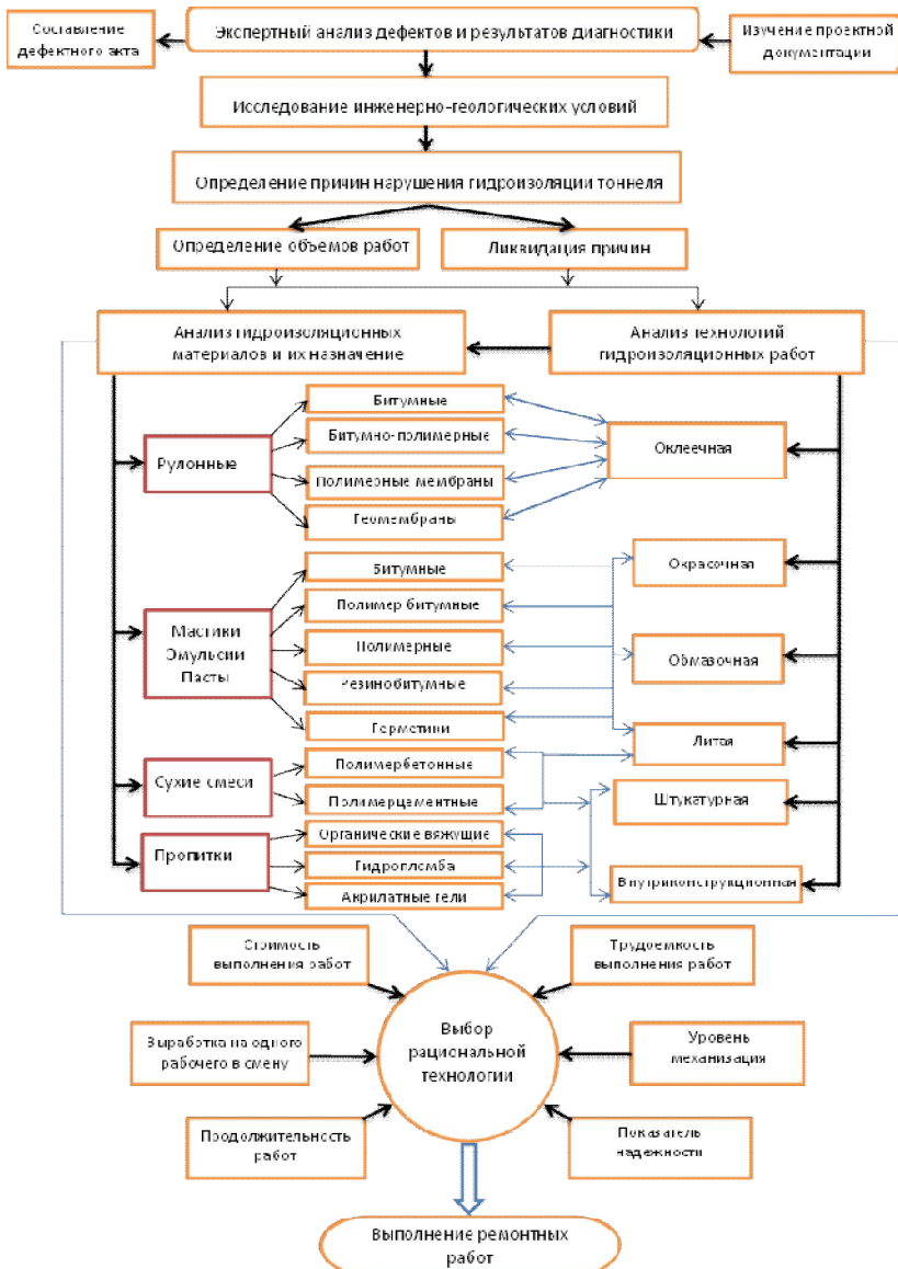
Рис.1. Блок-схема выбора технологии ремонта гидроизоляции тоннелей Данный алгоритм позволяет, при последовательном выполнении операций достичь окончательного результата, то есть выбрать
