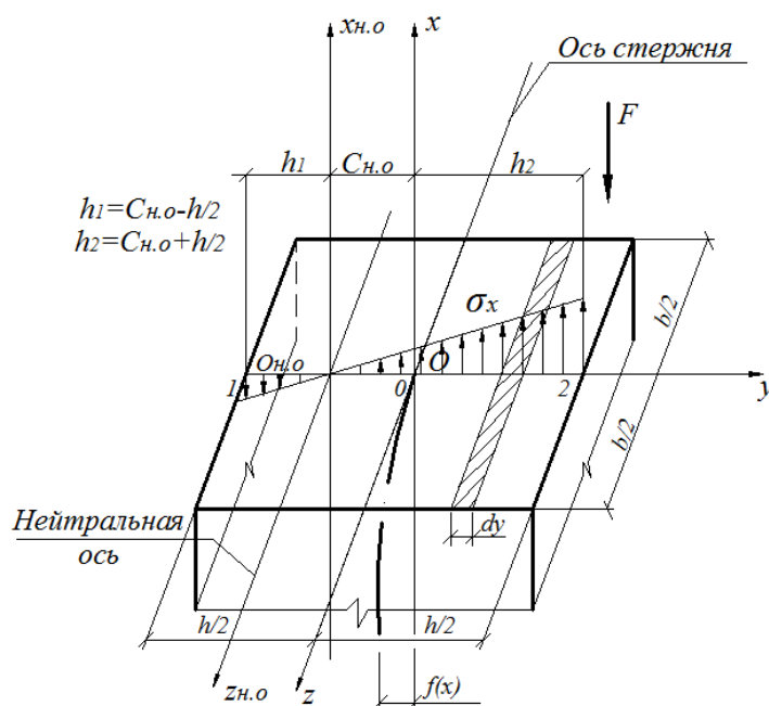
Рис. 3. Напряженное состояние при большом эксцентриситете
