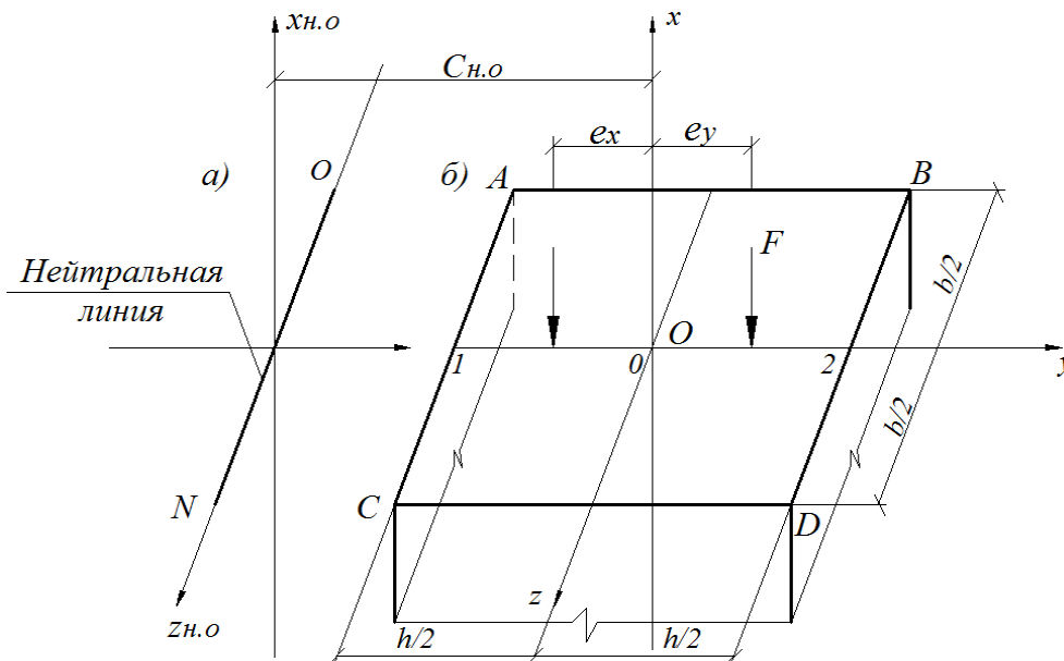
Рис. 1. Схема внецентренно сжатого стержня
