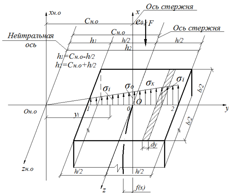
Рис. 2. Напряженное состояние при малом эксцентриситете
