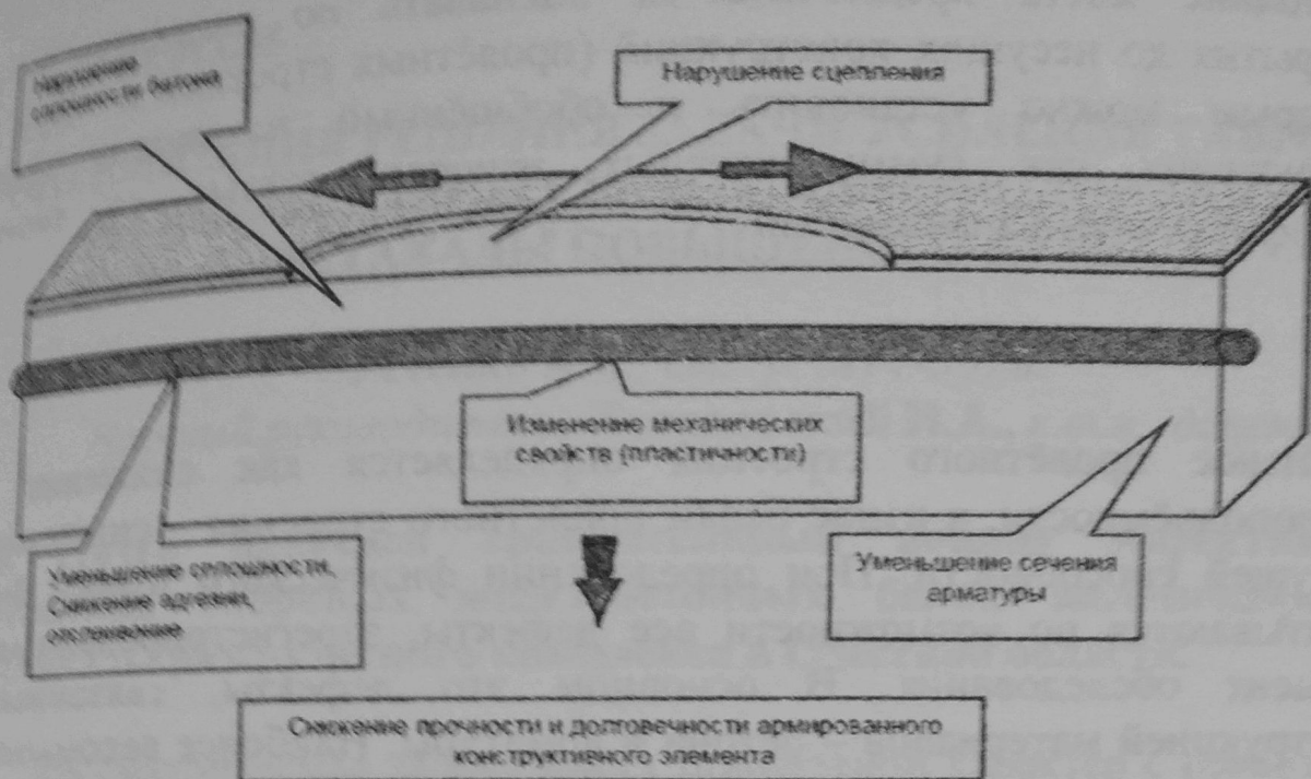
Рис. 3. Последствия коррозионного поражения железобетонной конструкции
