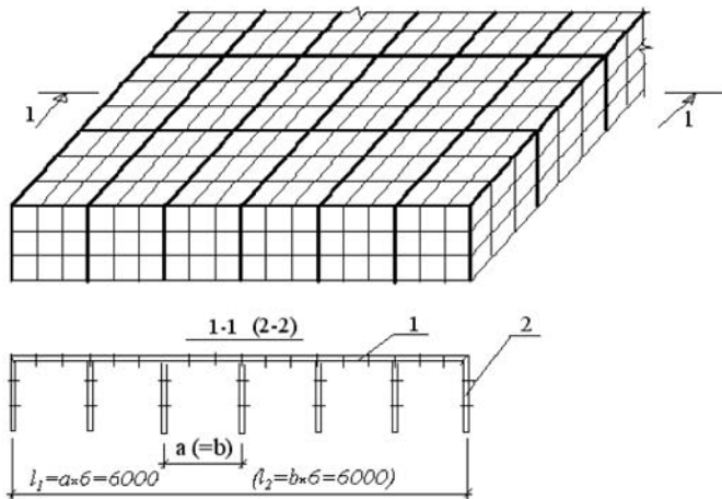
Рис. 1. Расчетная МКЭ-схема кессонного перекрытия при представлении полок и ребер плоскими конечными элементами: 1 – КЭ полки; 2 – КЭ ребер
