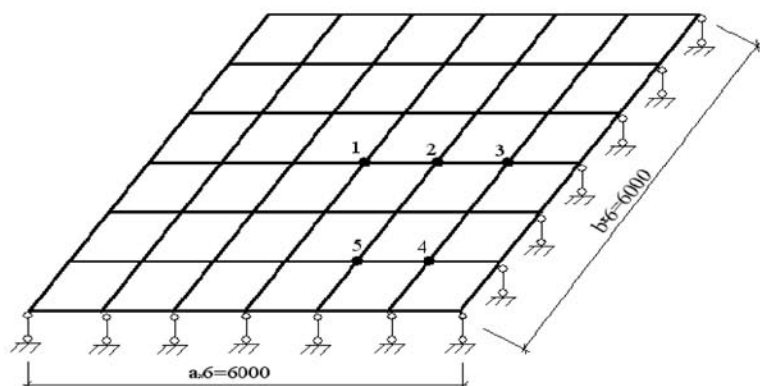
Рис. 2. Расчетная схема кессонного перекрытия в виде стержневой аппроксимации
