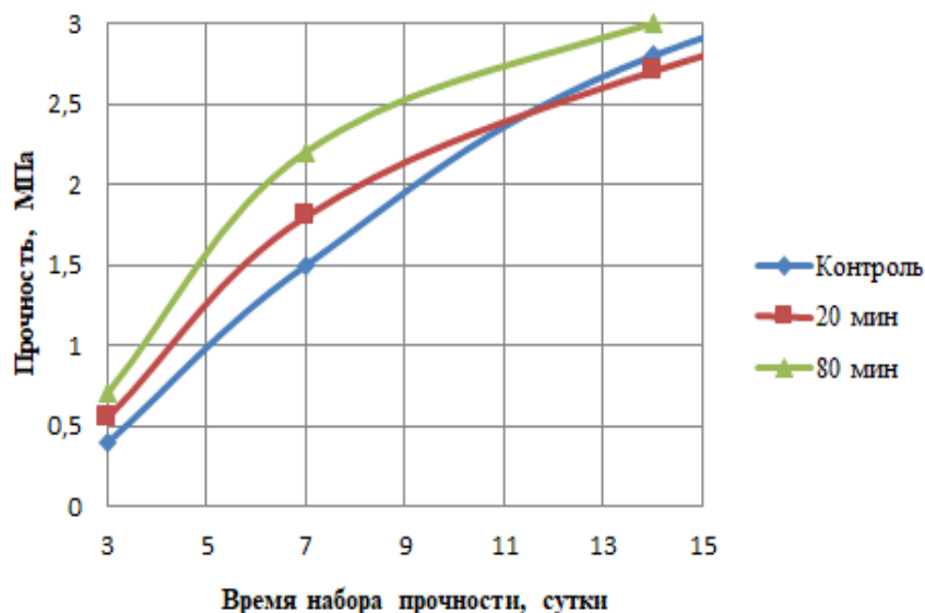
Рис. 1. Влияние акустической активации на прочность пенобетона
