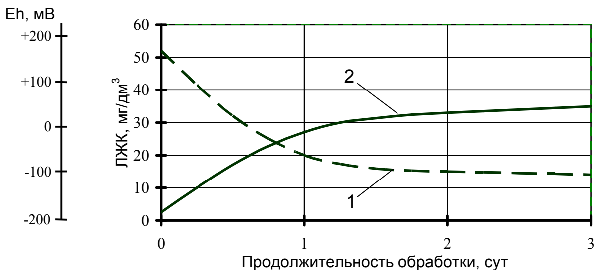
Рис. 2 – Зависимость окислительно-восстановительного потенциала Eh и концентрации ЛЖК от продолжительности обработки сточных вод в септике: 1 – изменение Eh; 2 – изменение ЛЖК
