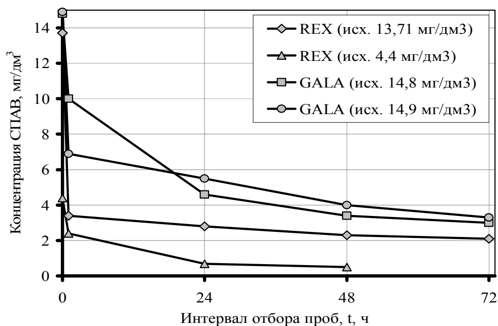
Рис. 1 – Зависимость концентрации СПАВ от продолжительности обработки сточных вод в септике
