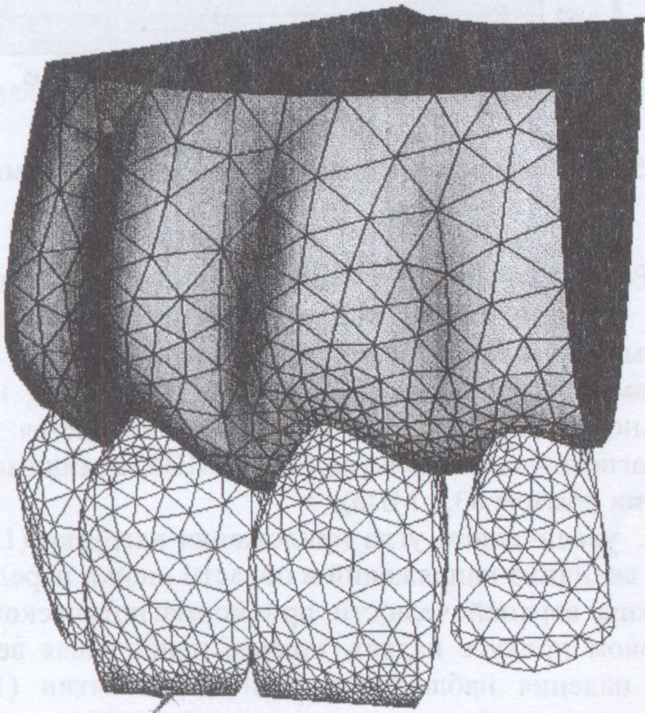
Рис. 1. Фрагмент модели зубочелюстной системы.
