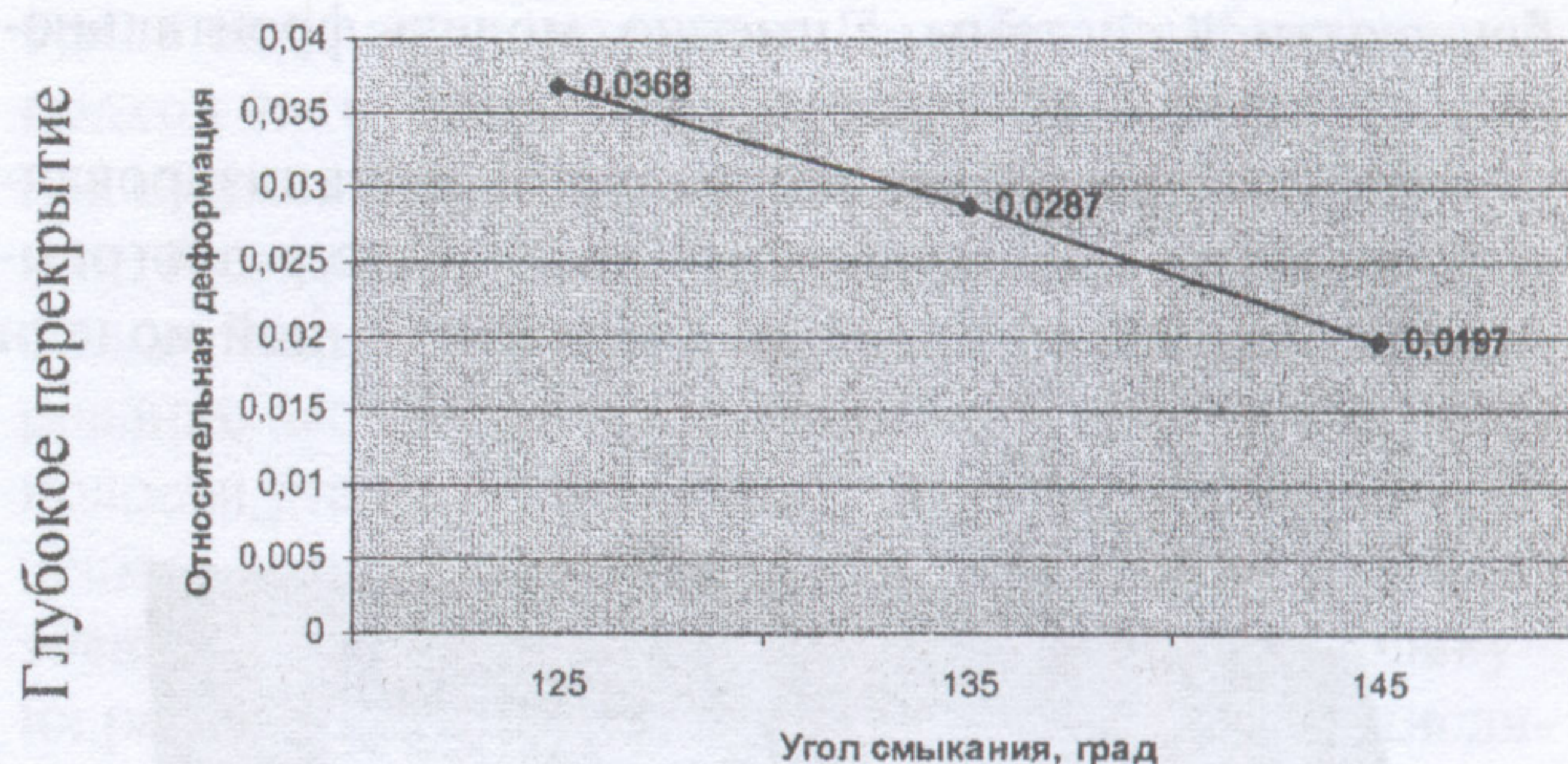
Рис. 5. Относительные деформации при трех типах смыкания.
