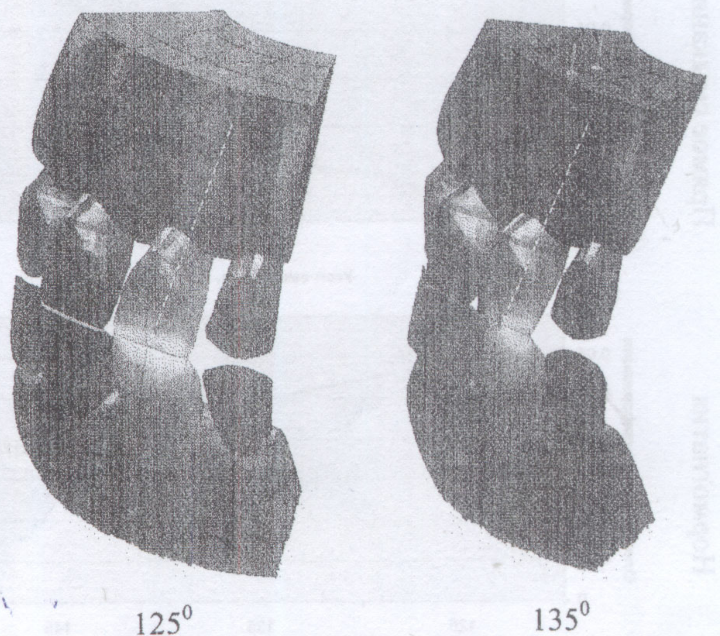
Рис. 3. Поля напряжений при прямом смыкании
