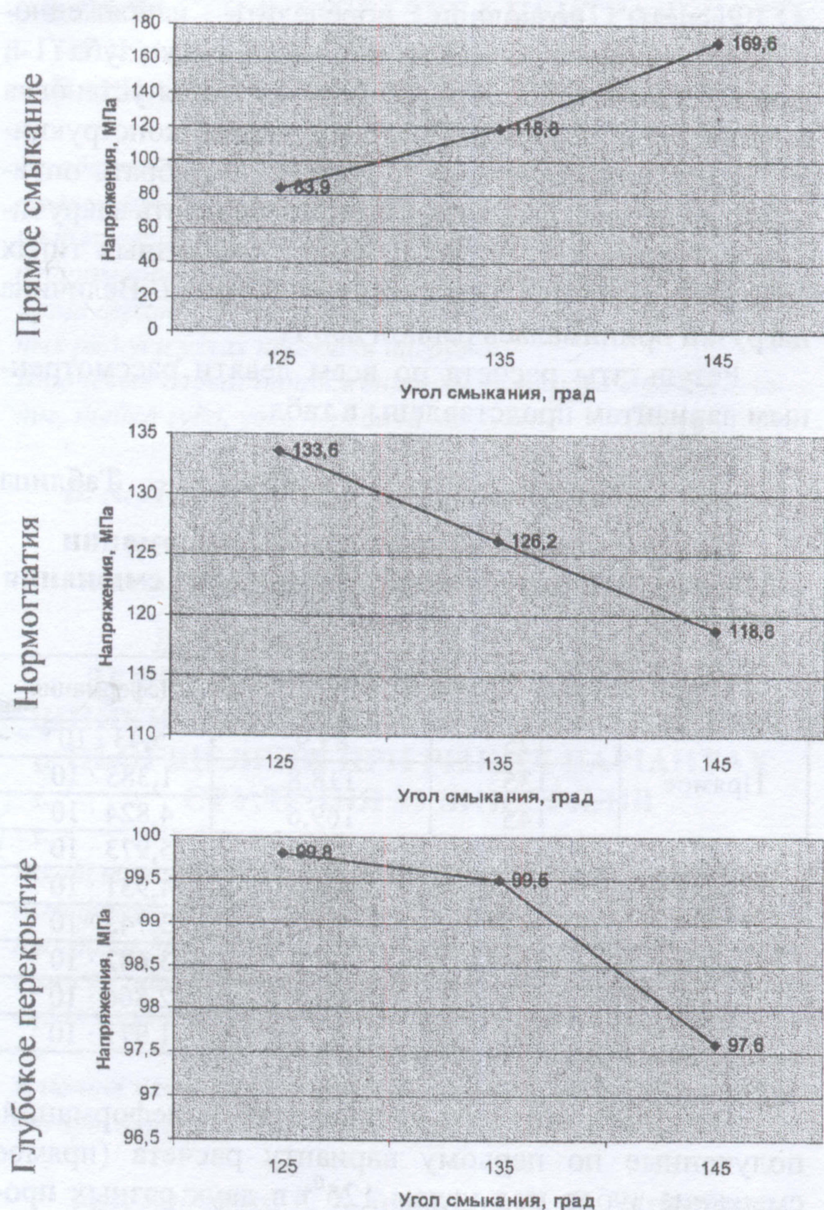
Рис. 4. Напряжения при трех типах смыкания
