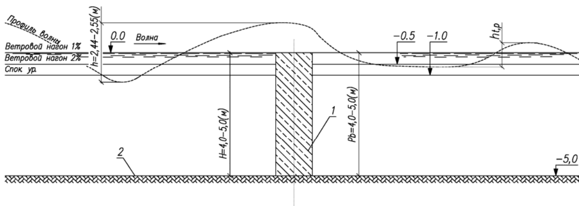
Рис. 3. Расчетная схема конструкции оградительного сооружения неполного профиля:
