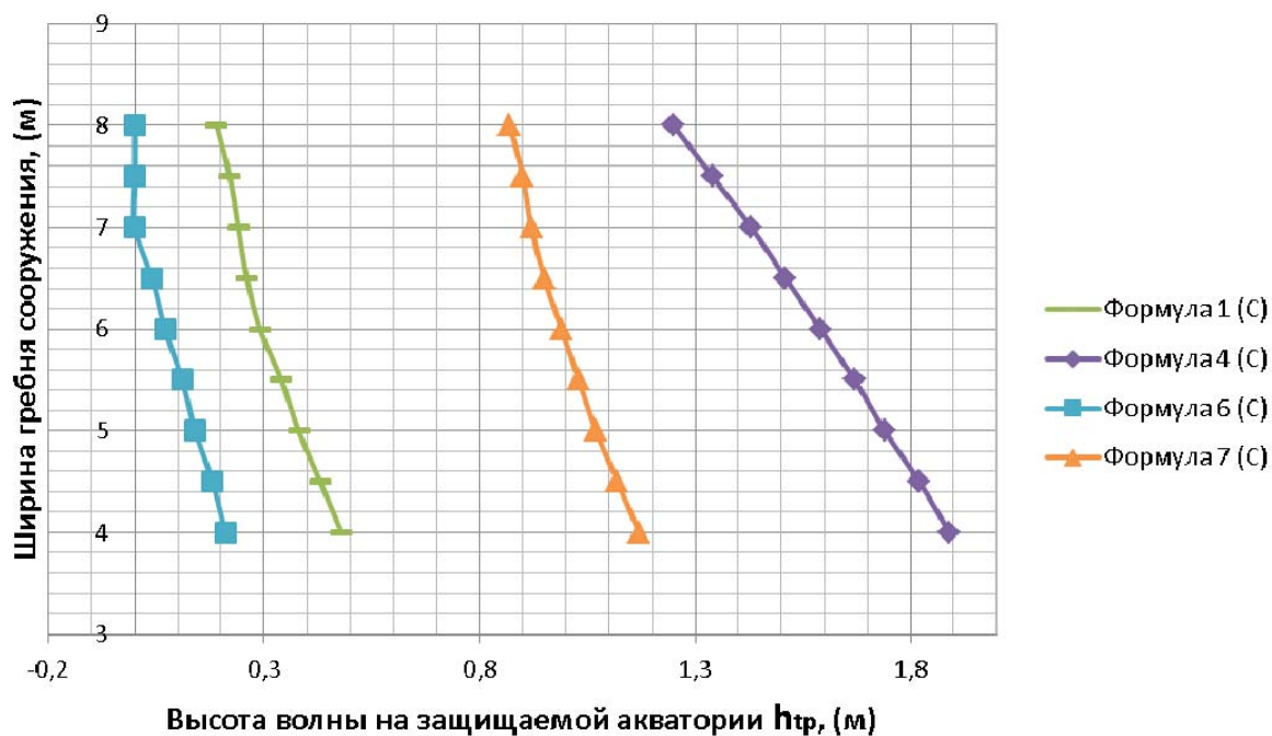
Рис. 6. График сравнения параметров трансформированных волн определенных различными методиками при расчетном случае (С)
