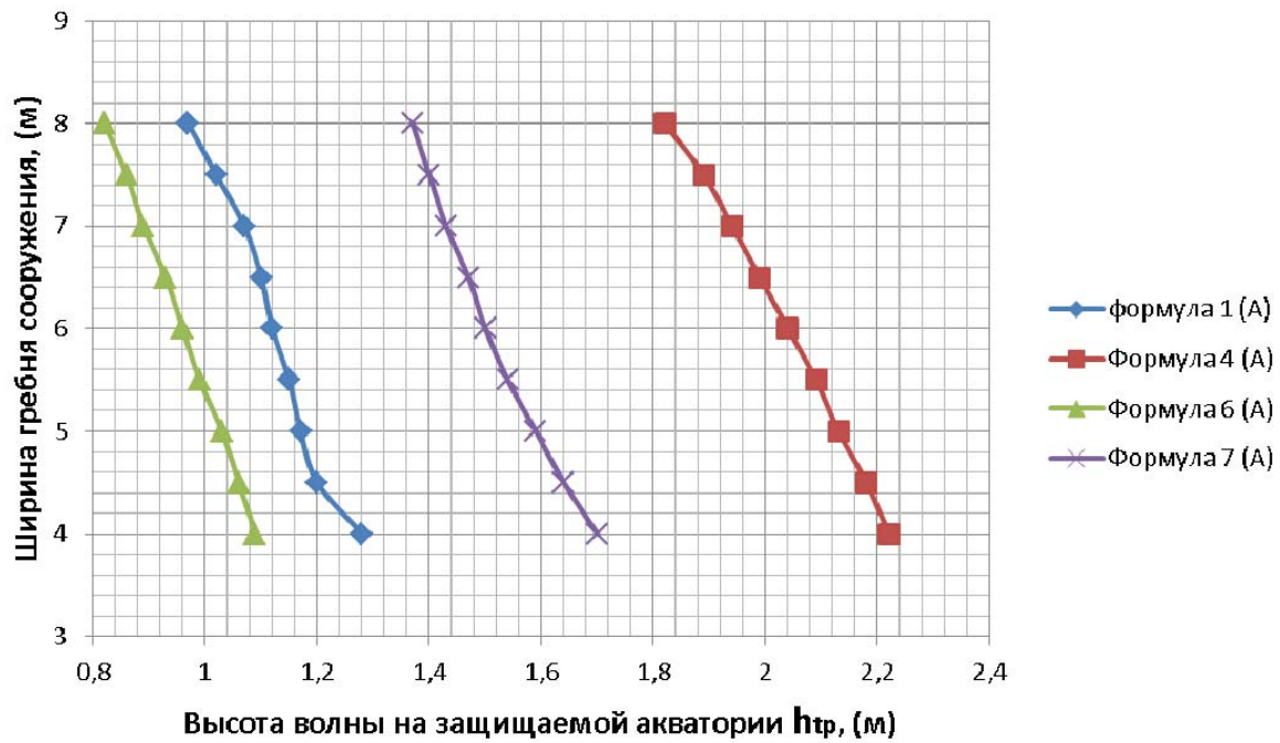
Рис. 4. График сравнения параметров трансформированных волн определенных различными методиками при расчетном случае (А)
