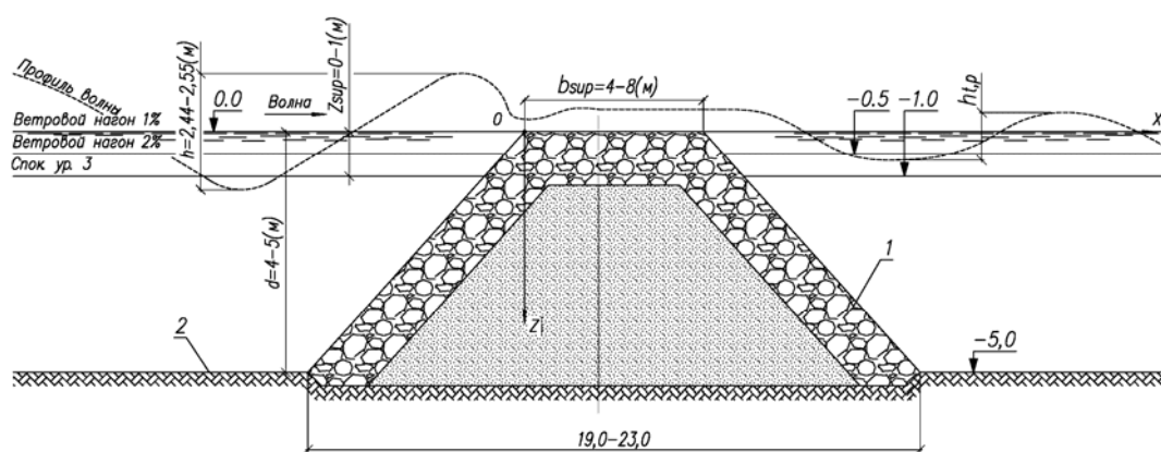
Рис. 2. Расчетная схема конструкции оградительного сооружения неполного профиля:
