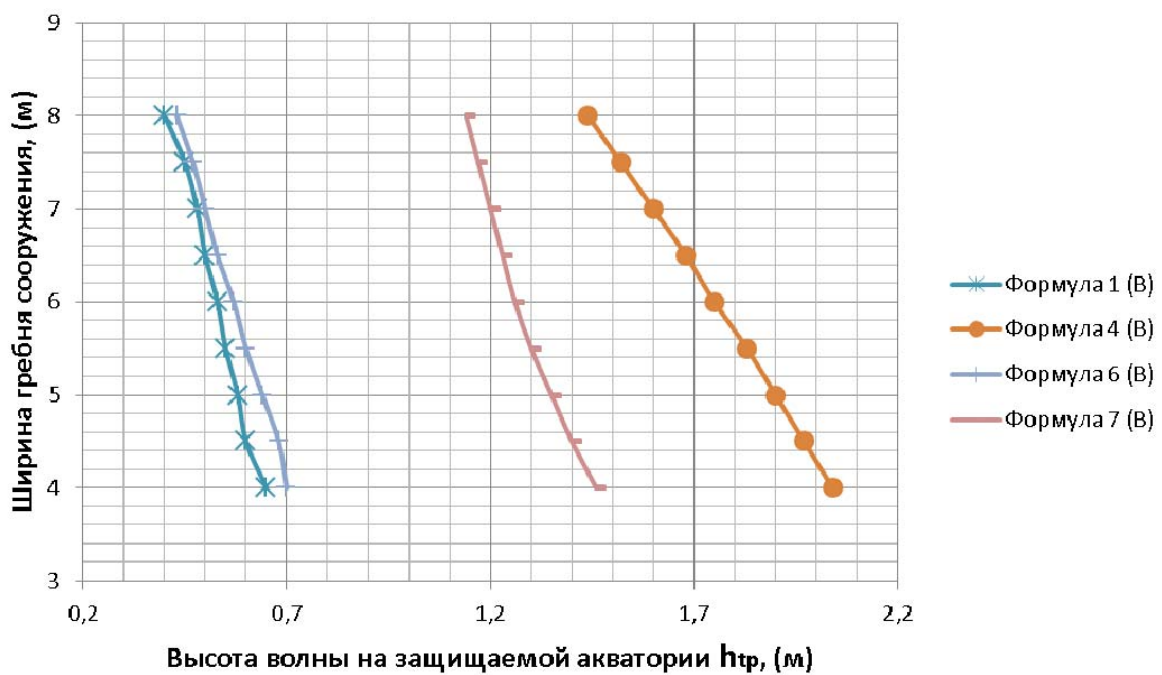
Рис. 5. График сравнения параметров трансформированных волн определенных различными методиками при расчетном случае (В)
