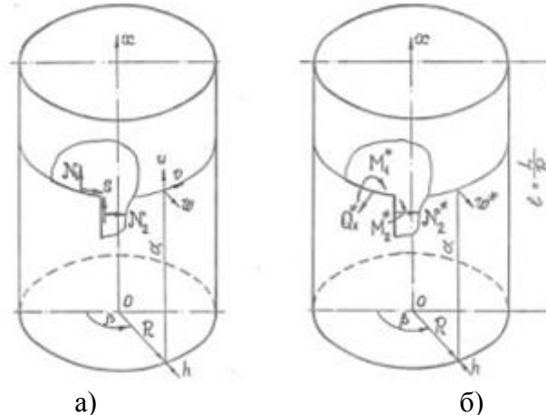
Рис. 2. Положительные направления усилий и перемещений: а – безмоментное напряженно-деформированное состояние; б – состояние краевого эффекта
