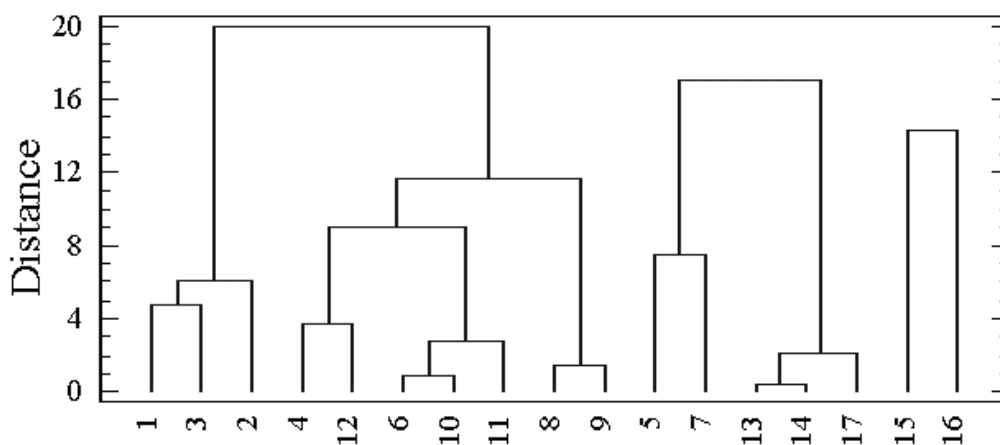
Рис. 4. Дендрограмма кластерного анализа
