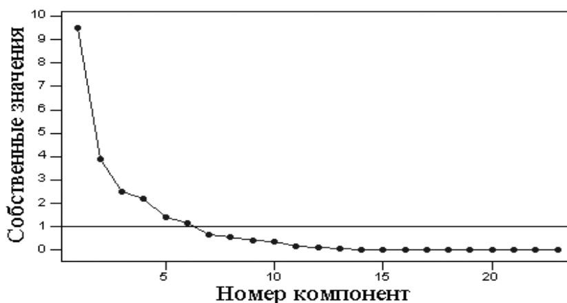
Рис. 3. Исследование собственных значений корреляционной матрицы
