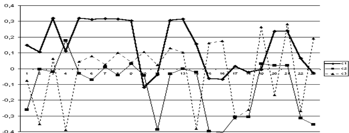
Рис.2. Коэффициенты первых трех главных компонент c1, c2, c3
