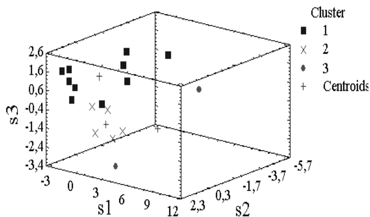
Рис. 5. Структура кластерів і групування результатів аналізу (S1, S2, S3 – три найбільш суттєвих комбінованих показателя)
