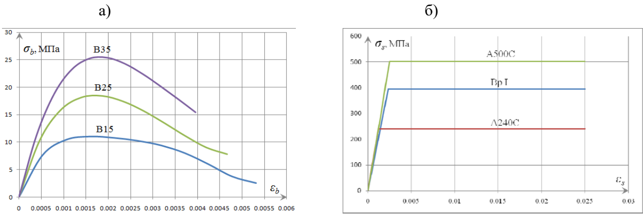
Рис. 1 – Діаграми деформування матеріалів: а) бетону; б) арматури
