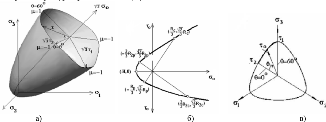
Рис. 2 – Фрагмент поверхні міцності бетону (а).
