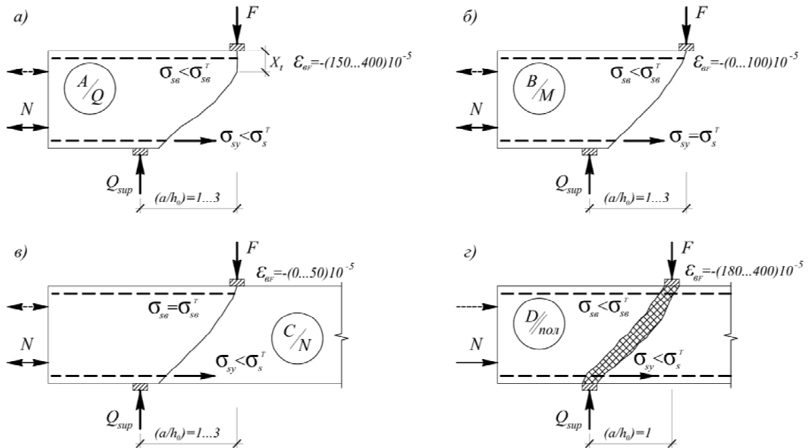
Рис.5. Можливі схеми руйнування припорних ділянок позцентрово розтягнутих або стиснутих залізобетонних балок від переважної дії поперечної сили (а), згинального моменту (б), поздовжньої сили (в), за похилою стислою смугою (г).
