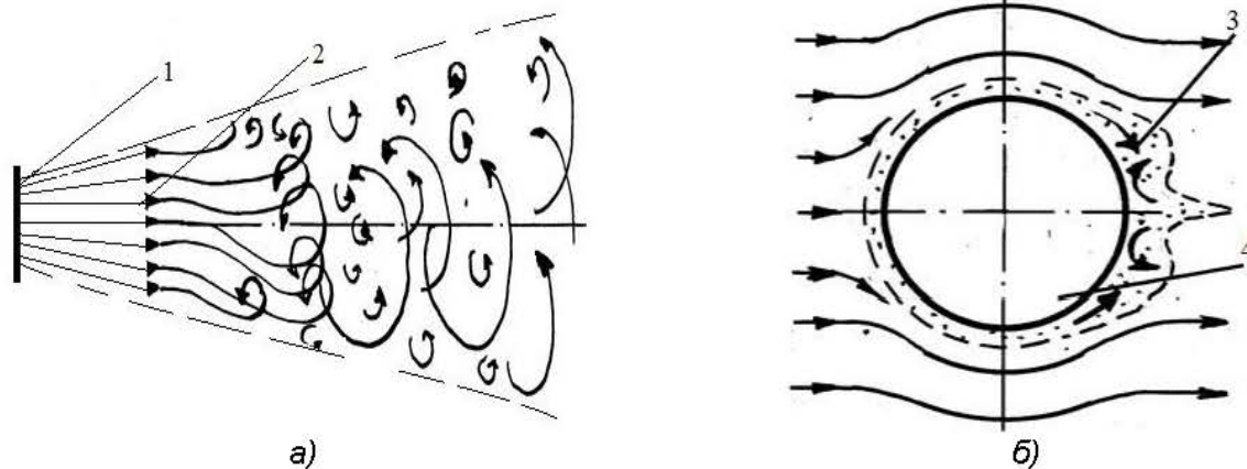
Рис. 2. Схеми виникнення турбулентного потоку при виході струменю з отвору ін'єктора (а), за частиною ґрунта (б)
