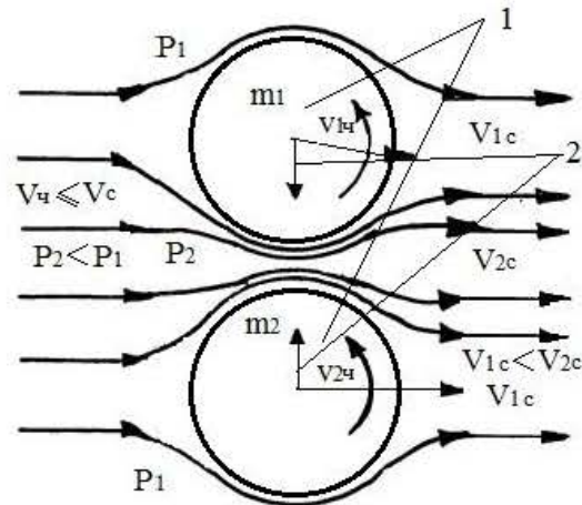
Рис. 1. Схема взаємодії часток в турбулентному потоці при їх русі сусідніх потоків: 1 – частинки ґрунту; 2 – сили гідродинамічного притягування часток; V_c – середня швидкість потоку; V_1, V_2 – абсолютні швидкості вихрових "ниток"; m_1, m_2 – маса частинок; P_1, P_2 – тиск
