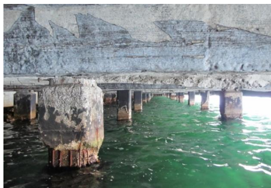
Рис. 3. Повреждения свайного основания
