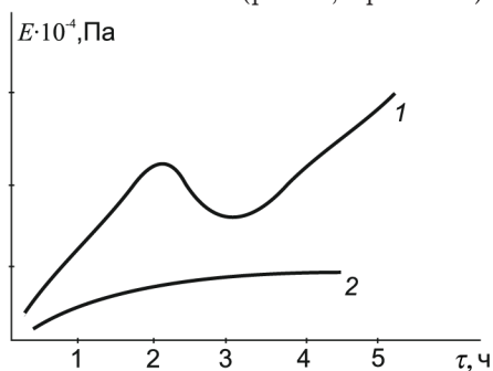
Рис. 1. Кривые изменения во времени t модуля быстрой эластической деформации E суспензии MgO: 1 – без поверхностно-активного вещества; 2 – с 1% содержанием лимонной кислоты
