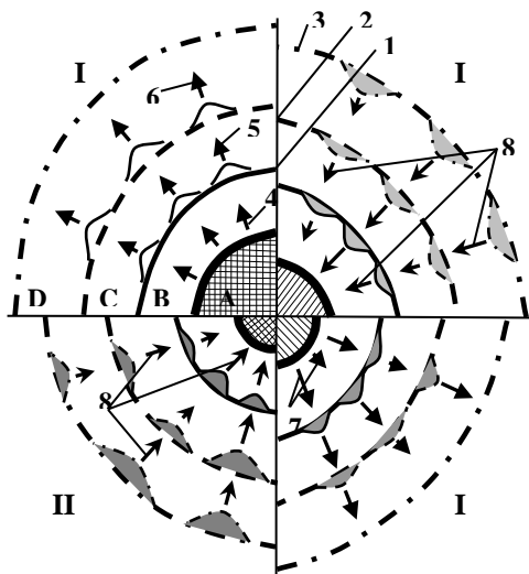
Рис.1. Схема развития собственных деформационных процессов в период организации структуры бетона как сложноорганизованного материала:
