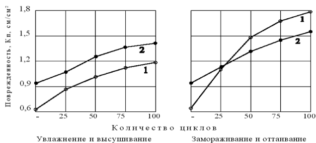
Рис.2. Изменение поврежденности в условиях малоциклового эксплуатационного воздействия:
