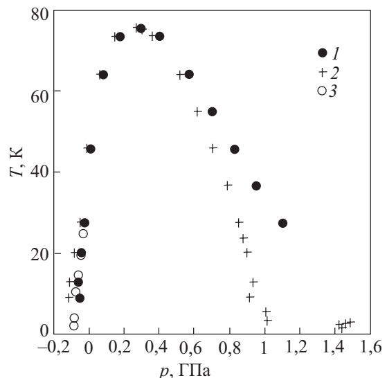
Рис. 3. Рассчитанная линия спинодали ГЦК Ne (1) с учетом квантового вклада (24) (для сравнения символами 2 показана «универсальная» линия спинодали [18] для кристаллов типа Ar). 3 — данные компьютерных «экспериментов» для Ne [22].
