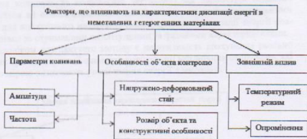
Рис. 1. Фактори, що впливають на дисипативні властивості виробів із неметалевих гетерогенних матеріалів
