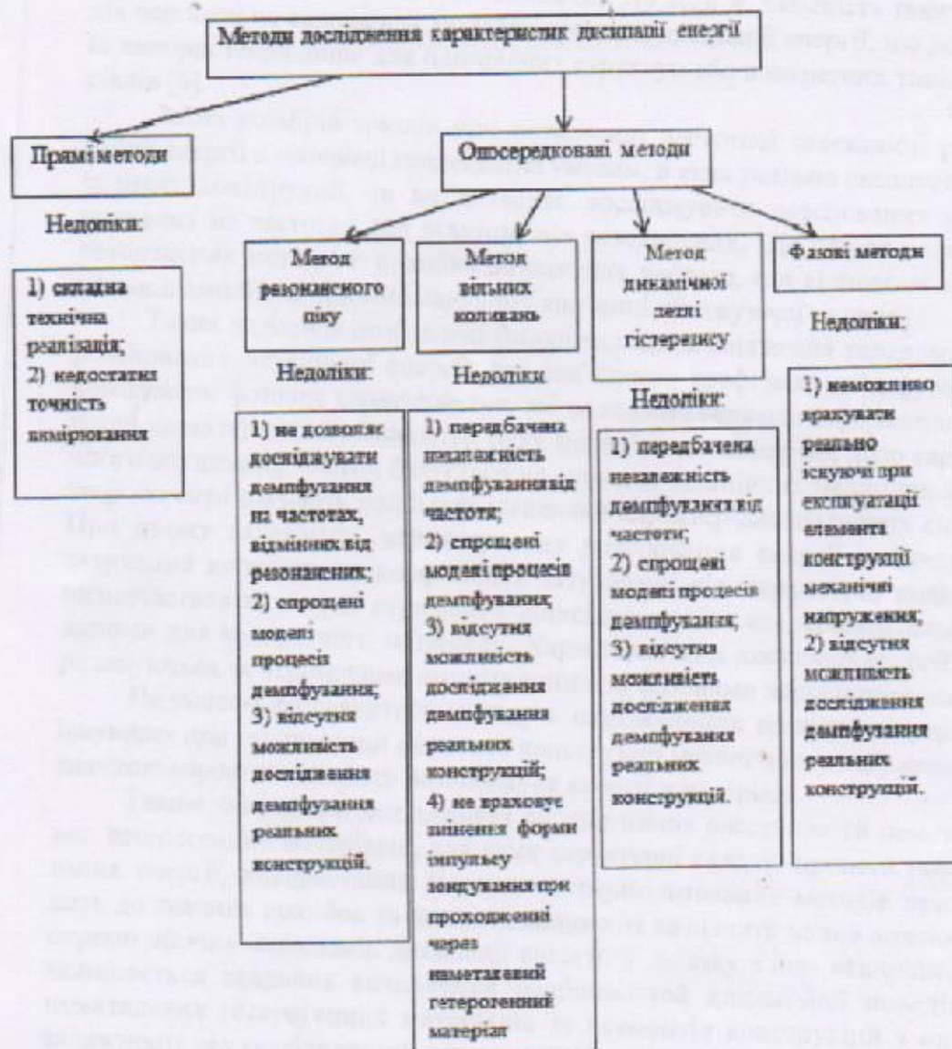
Рис. 2. Методи дослідження дисипативних властивостей матеріалів
