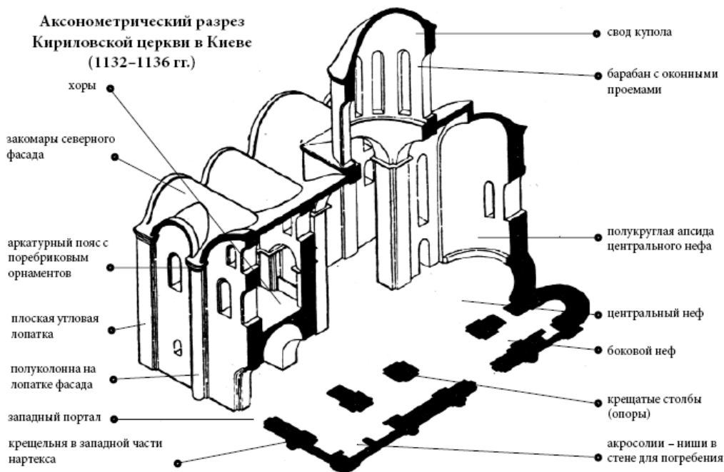
Рис. 8. Объемно-планировочное построение православных храмов Киевского княжества середины XII в. (30–80-е гг.) и их характерные черты
