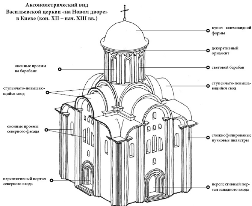
Рис. 12. Объемно-планировочное построение православных храмов Киевского княжества конца XII – пер. пол. XIII вв. и их характерные черты
