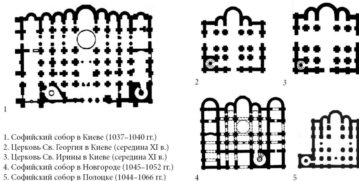
Рис. 1. Планировка храмов Киевского государства первой половины XI в.
