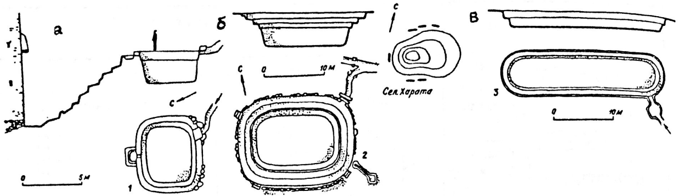
1. Джабии – бассейны для сбора и хранения воды. Планы, разрезы: а – в сел. Хурейхар (вади Дауан); б – в сел. Мешед (вади Дауан); в – возле сел. Харата (вади Духр) – по Ю.Ф.Кожину
