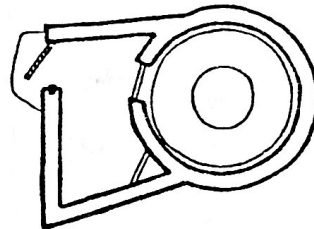
3. Вади Дуан. Небольшие джабии, перекрытые уполами возле сел. Хаджарейн: 1- Колодец; 2-сикая; 3-джабия с куполом. (по Ю.Ф.Кожину)
