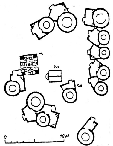
3. Вади Дуан. Небольшие джабии, перекрытые уполами возле сел. Хаджарейн: 1- Колодец; 2-сикая; 3-джабия с куполом. (по Ю.Ф.Кожину)
