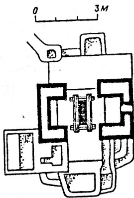
2. Вади аль-Каср. Колодец возле усадьбы ар-Рауда (по Ю.Ф.Кожину)
