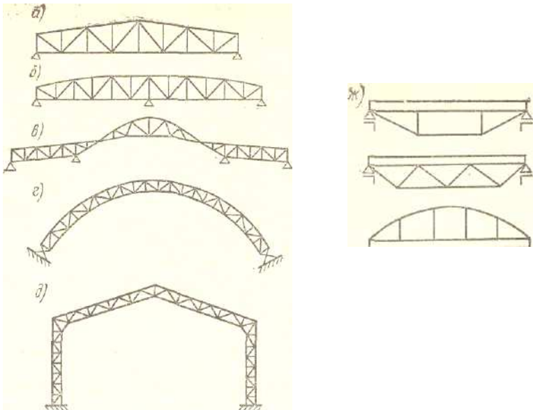
Рис.1. Системи ферм.
