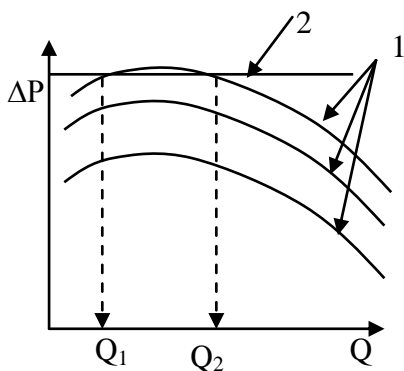
Рис.1 Характеристика нагнетателя Н1200 (1) и воздуховодка (2)
