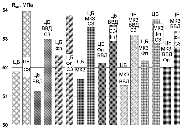
Рис. 3 Зависимость прочности R_{сж} (образца 10x10x10) от величины, введенной в его состав добавок: СП - С3, микрокремнезема - МКЗ, воздухововлекающей добавки РТ-1 - ВВД, полипропиленовой фибры - Фп
