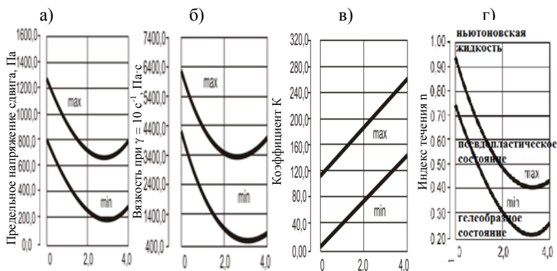
Рис.2. Влияние РДП на предельное напряжение сдвига (а) и вязкости при скорости деформаций \dot{\gamma} = 10 \text{ с}^{-1} (б), а также коэффициент K (в) и индекс течения n (г)
