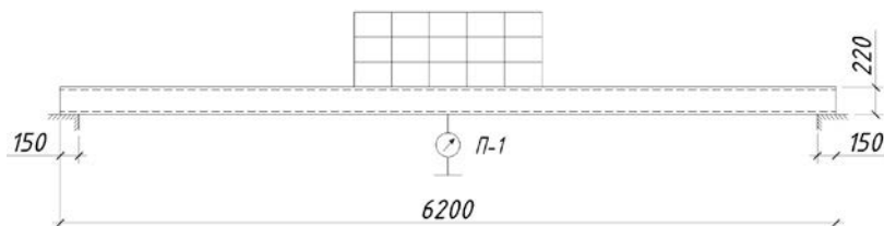
Рис.4. Схема испытания плиты покрытия нагрузкой
