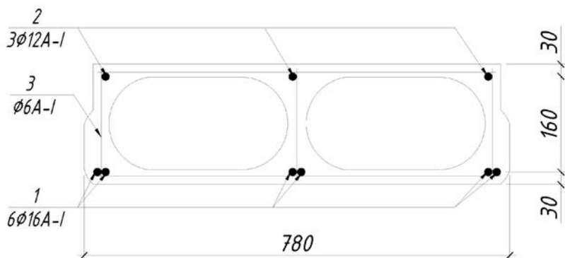
Рис.2. Сечение плиты
