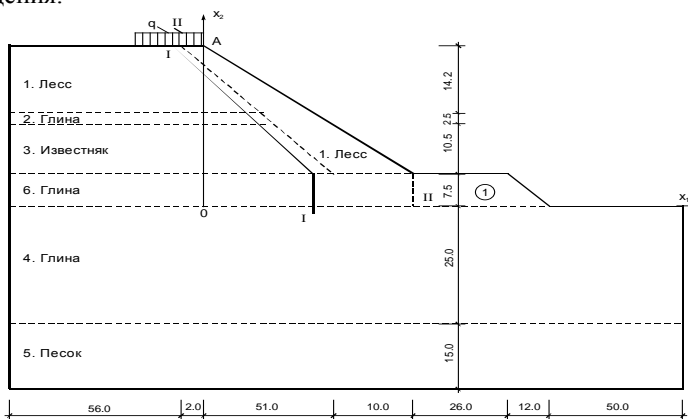
Рис. 1. Расчетная схема спланированного откоса
