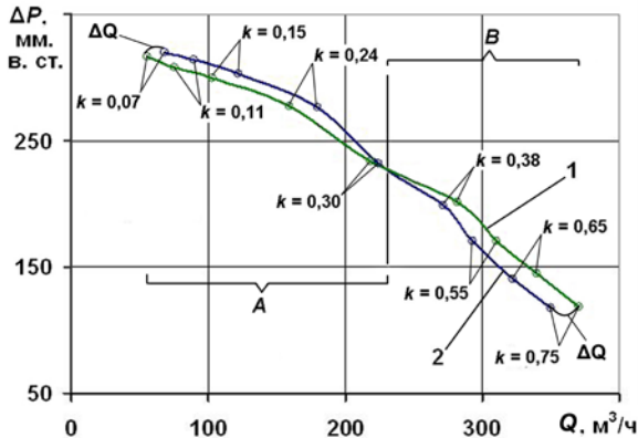
Рис. 5. Напорные характеристики вентилятора 1 – диафрагма – сопротивление установлена на стороне разряжения; 2 – диафрагма – сопротивление установлена на стороне давления
