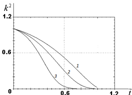
Рис. 2. Графики изменений квадрата модуля эллиптических функций для твердого тела в среде с сопротивлением
