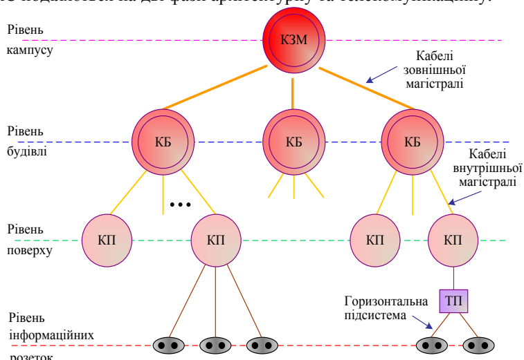
Рисунок 1. Схема структуризації кабельної системи: КЗМ - крос зовнішніх магистралей; КБ - крос будівель; КП - крос поверхів; ТП - точки переходу (необов'язково)
