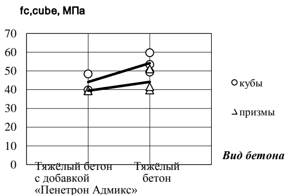
Рис.2. Распределение средних значений кубиковой и призмной прочности в зависимости от вида бетона.
