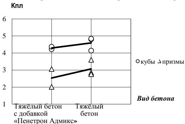
Рис.1. Распределение средних значений коэффициентов повреждённости кубов и призм в зависимости от вида бетона
