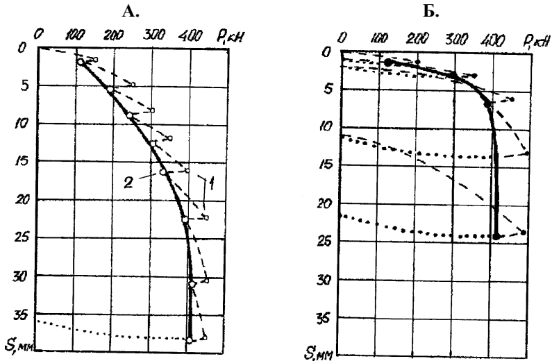
Рис. 5. - Результаты испытаний сваи № 2:
