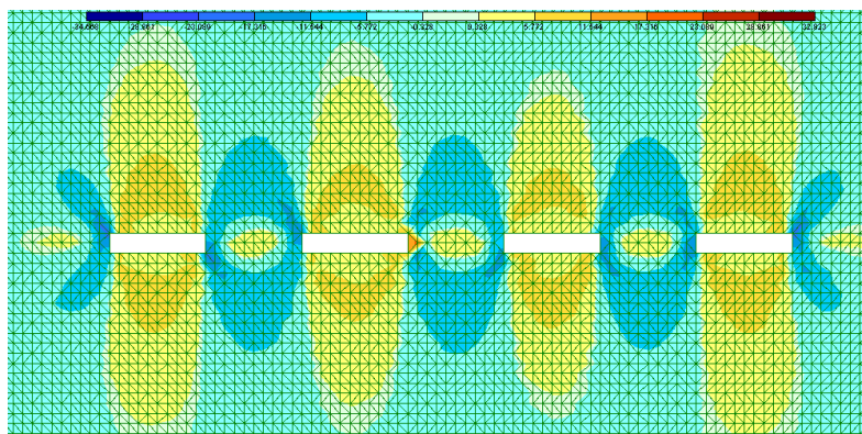
Рис.3. Напряжения N_{ув} области непровара
