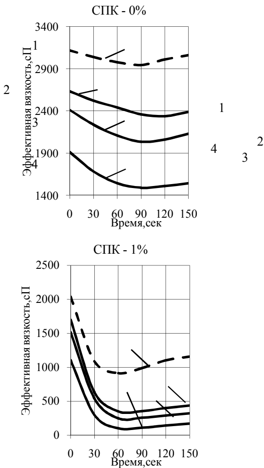
Рис 1. Влияние времени механоактивации на изменение эффективной вязкости цементосодержащей суспензии: 1; 2; 3; 4 – содержание доменного шлака в портландцементе соответственно 0%; 30%; 45%; 60%
