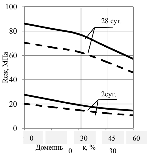
Рис.2. Влияние содержания доменного шлака в вяжущем на R_{сж} цементного камня
