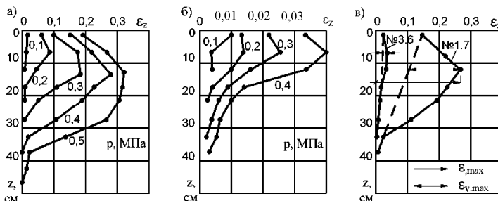
Рис. 7. Изменение эпюр относительных послойных деформаций по глубине с увеличением давления в опытах № 1.7 (а) и № 3.6 (б); в) – то же, при давлении 0,4 МПа по подошве штампа в опытах №№ 1.7 и 3.6.
