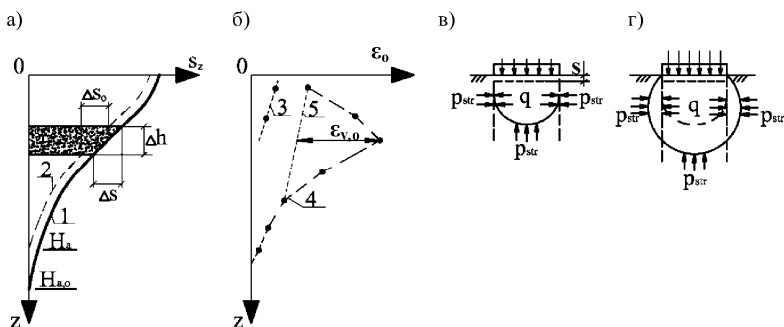
Рис.3. Эпюры: а) – полных (1) и остаточных (2) деформаций по глубине основания; б) – относительных значений остаточных деформаций: (3) – при q \leq p_{str} ; (4) – при q > p_{str} ; в) и г) – схемы деформирования грунта при: q \leq p_{str} и q > p_{str} , соответственно
