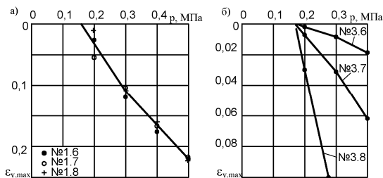
Рис. 8. Границы зависимости максимальных значений относительных деформаций от давления: а) – по результатам серии опытов
