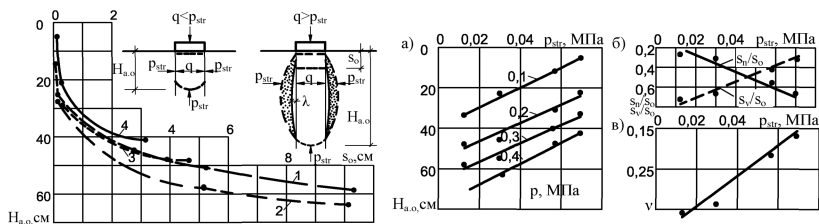
Рис. 2. Влияние структурной прочности на параметры напряженно-деформируемого состояния грунтов в основании штампа: а) – зависимость глубины зоны остаточных деформаций H_{a.o} от остаточной составляющей осадки s_0 ; б) – зависимость глубины зоны остаточных деформаций H_{a.o} от p_{str} ; в) – влияние p_{str} на соотношения осадок, вызванных уплотнением и поперечным расширением; г) – зависимость коэффициента поперечного расширения от p_{str} .
