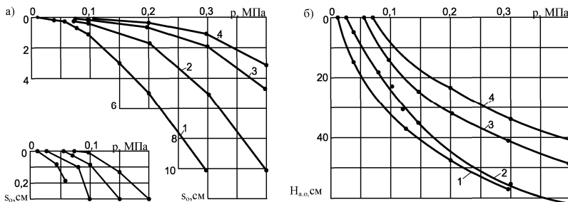
Рис. 1. Графики нарастания остаточных осадок s_0 (а) и глубины зоны остаточных деформаций H_{a.o} (б) от давления p (цифрами показаны номера опытов)
