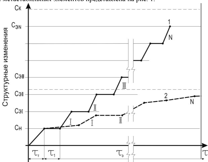
Рис. 1. Принципиальная схема взаимодействия активных и метастабильных элементов структуры материала в период эксплуатации конструкции: \tau_T , \tau_1 , \tau_3 – технологический, предэксплуатационный и эксплуатационный периоды жизни конструкции как открытой системы. C_N , C_{ЭI} , ... C_{ЭN} – начальные и эксплуатационные структурные изменения; C_K – критическое изменение структуры; I, II, ... N – периоды внешних воздействий на материал конструкции. 1 – изменения параметров активных элементов; 2 – изменения параметров метастабильных элементов
