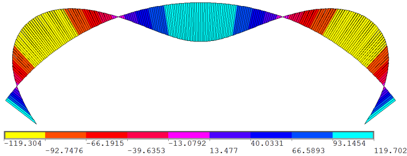
Рис. 9. Епюра згинальних моментів для безшарнірної арки постійної жорсткості у граничному стані при f/l = 0,25
