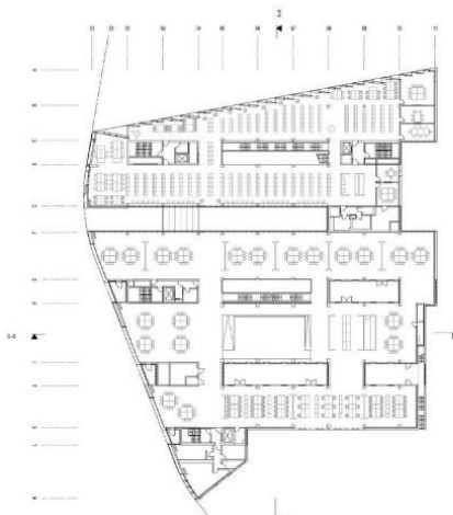
Рис. 1. Студія у Heneghan Peng Architects. Зліва: план першого поверху
