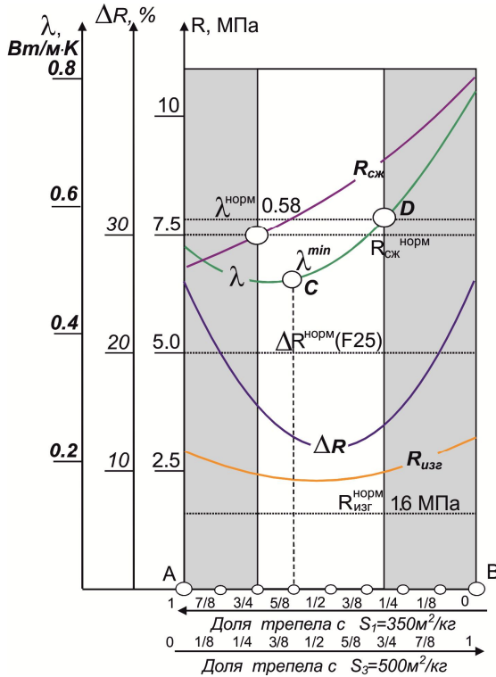
Рис. 2. Изменение свойств ССС (прочности при сжатии - R_{сж} , прочности на растяжение при изгибе - R_{изг} , коэффициента теплопроводности - \lambda , потери прочности при замораживании-оттаивании - \Delta R ) при изменении соотношения минерального наполнителя с различной удельной поверхностью
