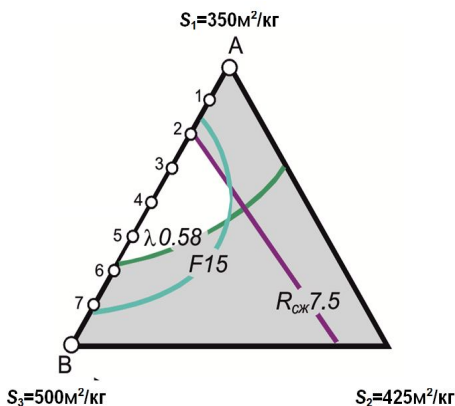
Рис. 1. Определение области оптимальной удельной поверхности наполнителя
