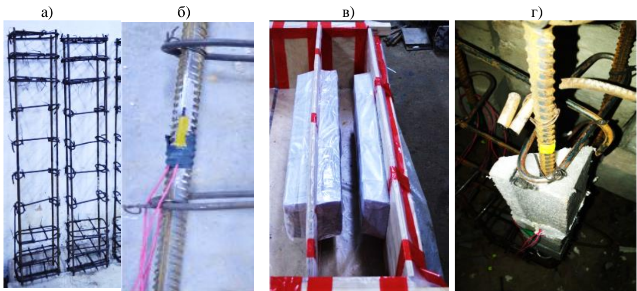
Рис. 3. Дослідні зразки: а – каркаси дослідних колон; б – тензодатчики; в – опалубка; г – моделювання пошкодження
