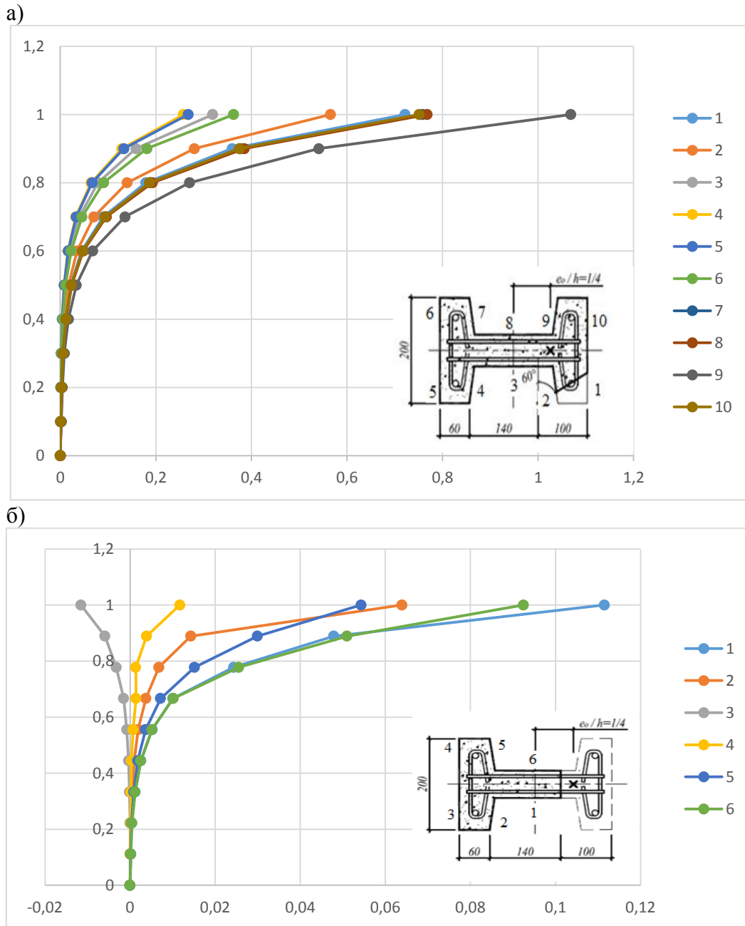
Рис. 6. Відносні деформації бетону та арматури ( \times 10^{-3} ): а – колони К 15; б – колони К 12
