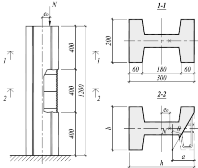
Рис. 4. Параметри дослідних зразків
