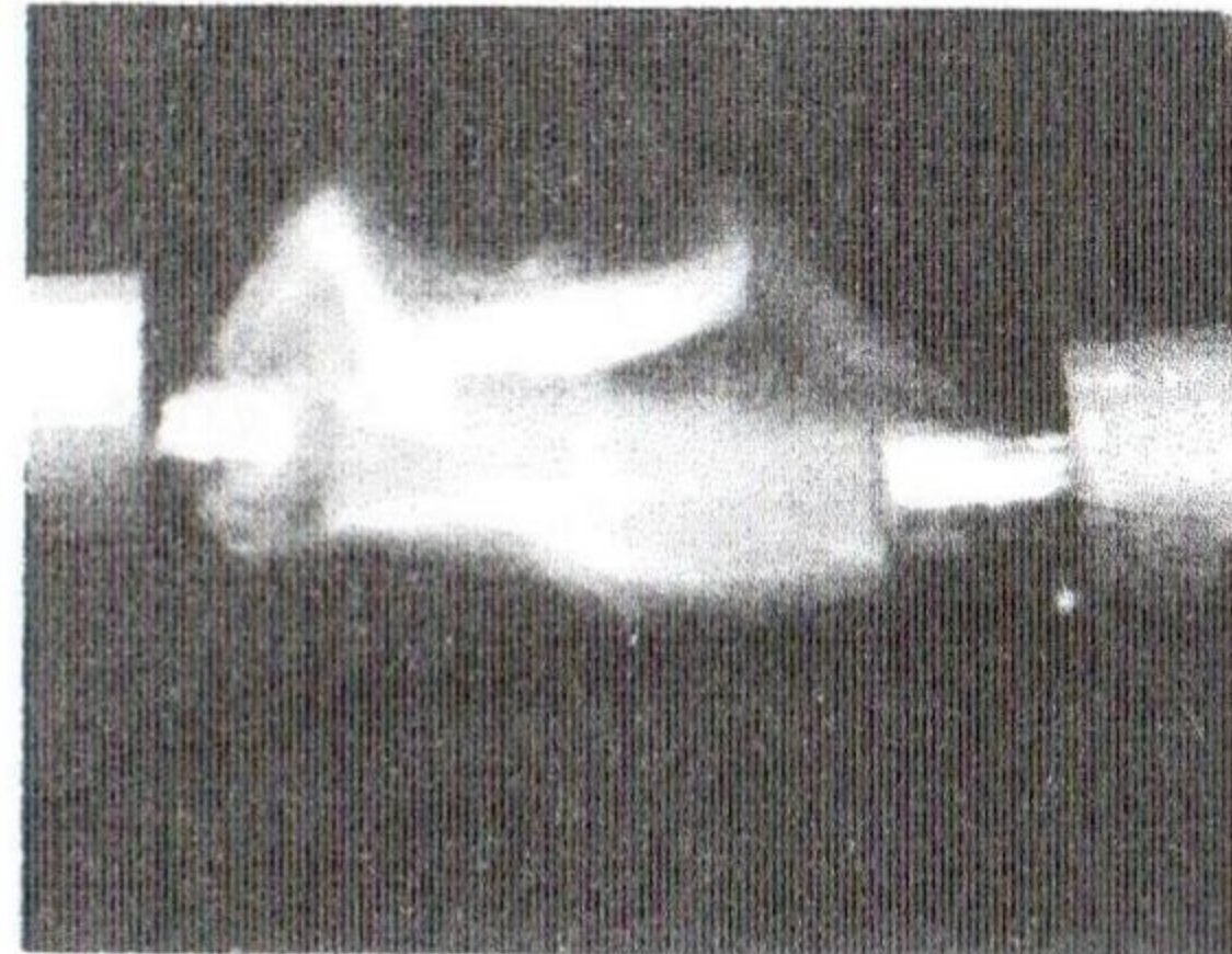
Рис.5. Взаимодействие встречных, смещенных в горизонтальной плоскости струй сжигаемого газа.
